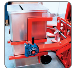
Logiflex met container (principe vatenkantelaar).
